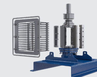
MÉCANISME DE COUPE DU PCM X-GUARD
