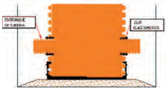
Finition du fond du regard avec base étanche (nécessaire avec nappe phréatique)
