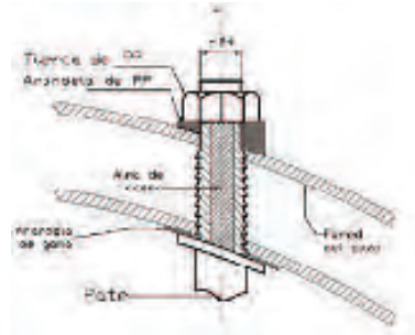
Détail de l'ancrage de l'échelon
