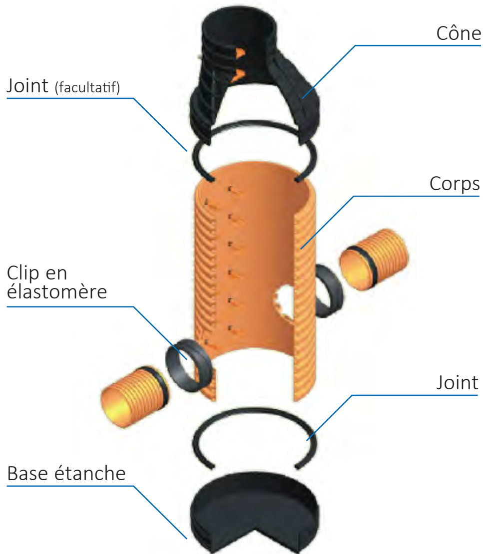
Schéma de la solution standard d'un regard SANECOR®.
