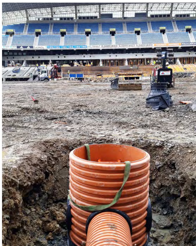
Réseau de drainage du terrain de football de Anoeta (San Sebastián)
