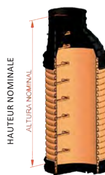
Regards D 1 000 et 1 200 mm
